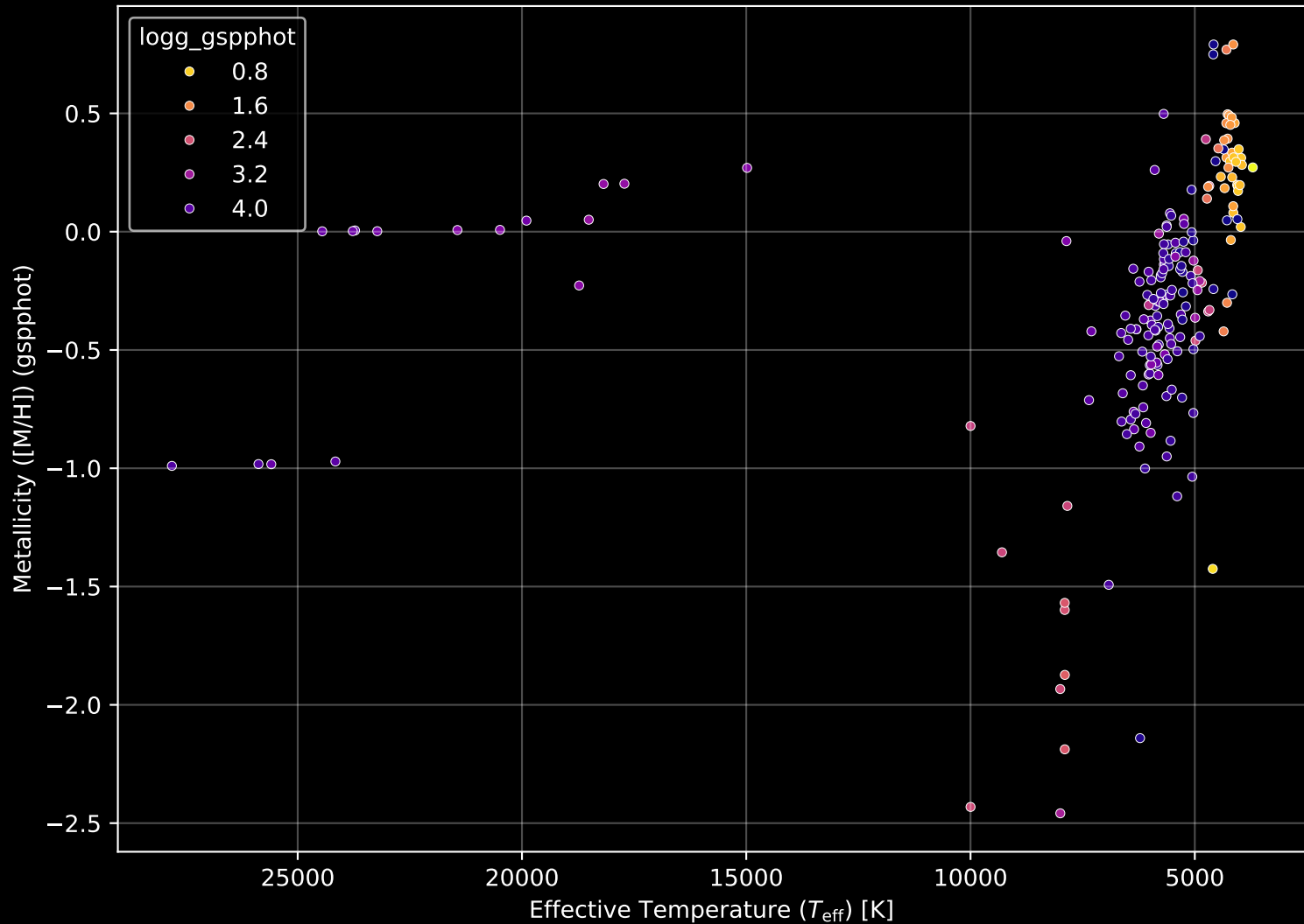
GALAH DR4 Field: [661] Stellar Population Parameters (n= 203)
